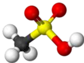
метансульфоновая
