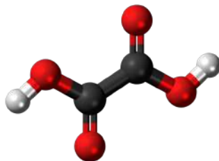
щавелевая
