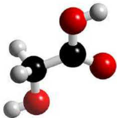
гликолевая
