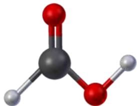
муравьиная
