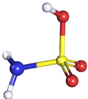
сульфаминовая
